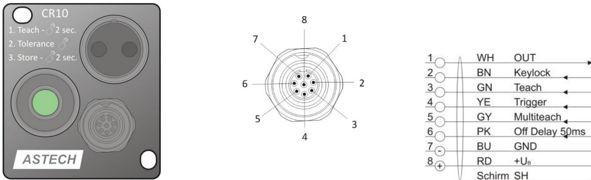
Abbildung 1 : Anschlusschema und Zählweise der Sensorbuchse
