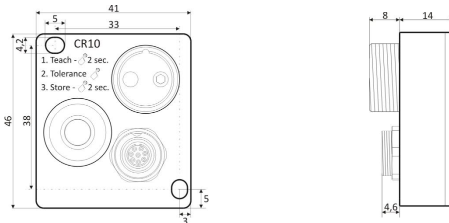
Abbildung 2 : Maßzeichnung CROMLAVIEW® CR10
