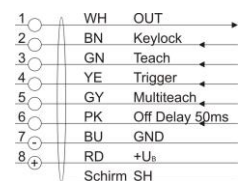
Anschlussschema
