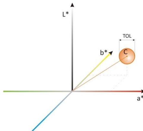
Abbildung 4 : Diagramm zur Erläuterung des Erkennungsmodus "Prüfen Kugeltoleranz"
